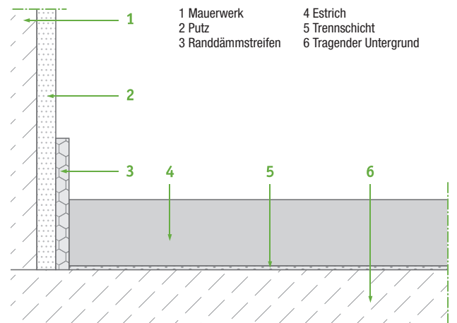
Abb. 4: Aufbau eines Estrichs auf Trennlage mit Planocem Zementestrich.
