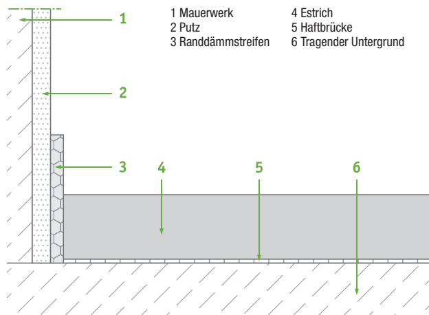
Abb. 3: Aufbau eines Verbundestrichs mit Planocem Zementestrich.
