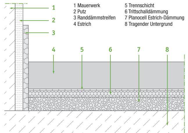
Abb. 2: Aufbau eines trittschalldämmten, schwimmenden Estrichs mit Planocem Zementestrich auf Planocell Estrich-Dämmung.
