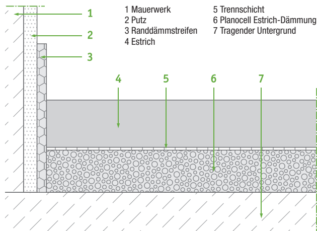
Abb. 1: Aufbau eines klassischen schwimmenden Estrichs mit Planocem Zementestrich auf Planocell Estrich-Dämmung.
